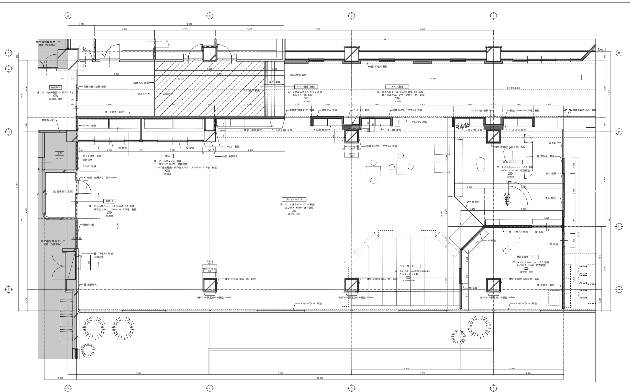
1階平面詳細図 2【改修】 SCALE 1:50
